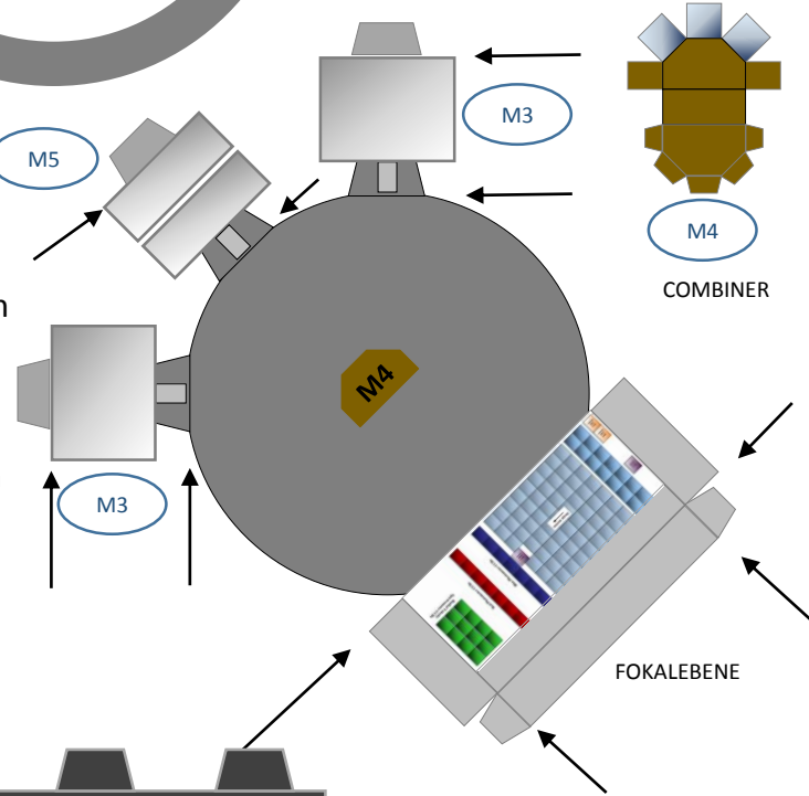
OPTISCHE BANK
